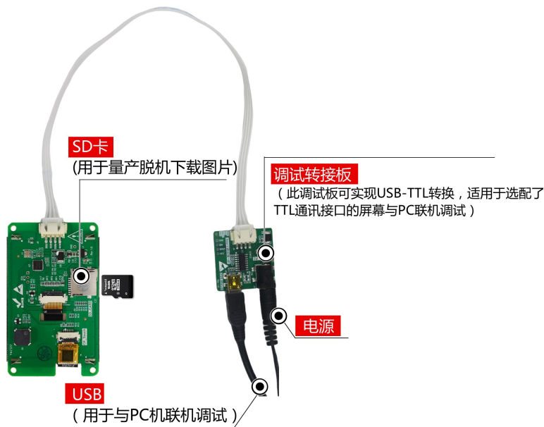
图 1-3 调试工具图
