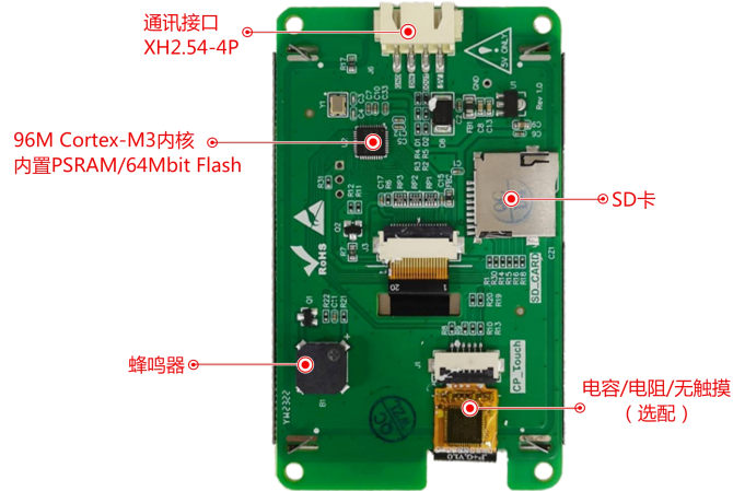
图 1-2 硬件配置图
