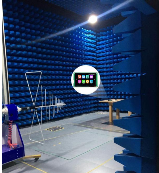
图 4-4 RE 测试图
